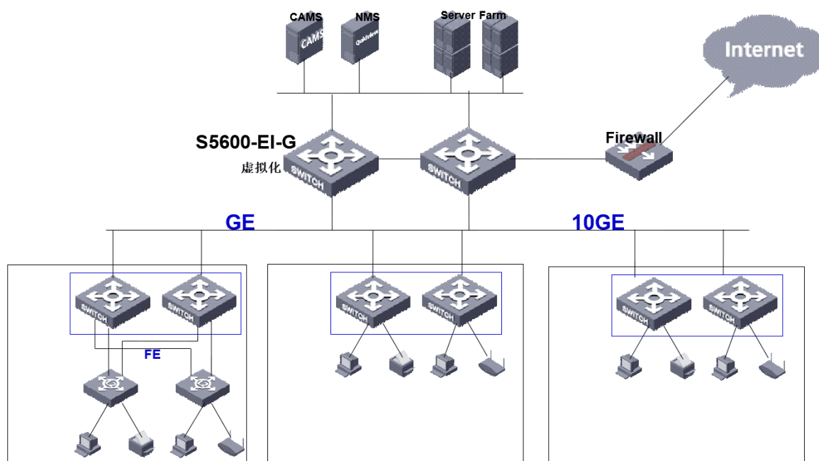
S5600-EI-G系列以太网交换机在核心层的应用
